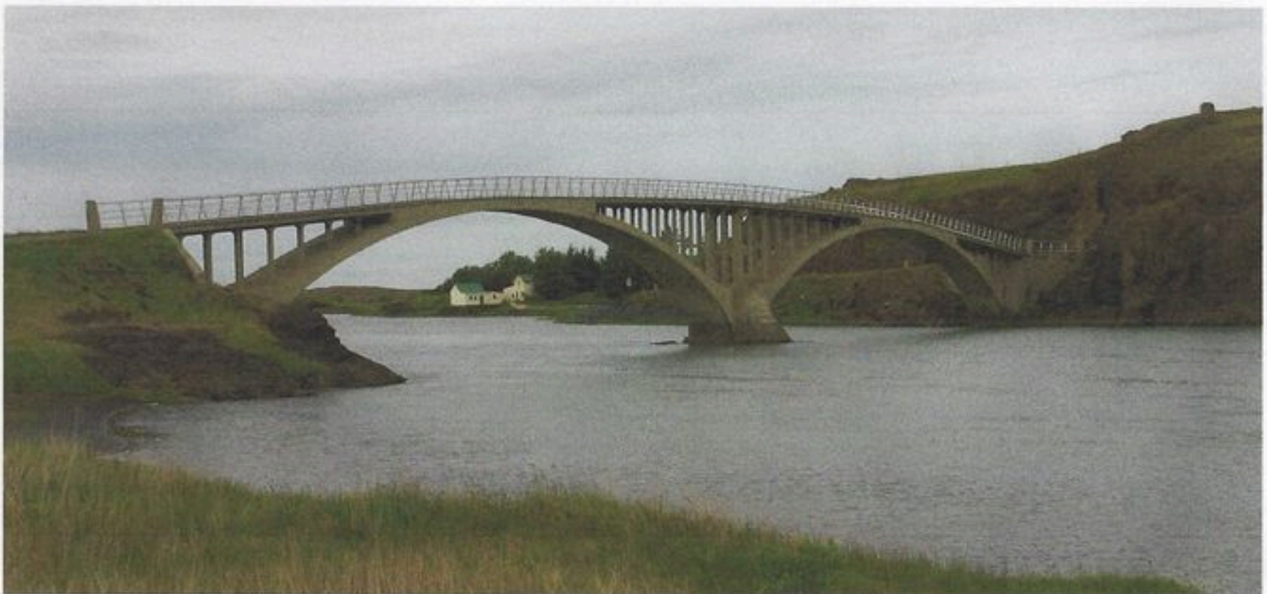
Hvita Hjúferjukoti - Island Stahlbetonbogenbrücke über die Hvita
